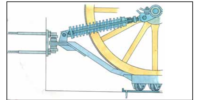
Med hjälp av en kraftig fjäder förankrades kanonen.
