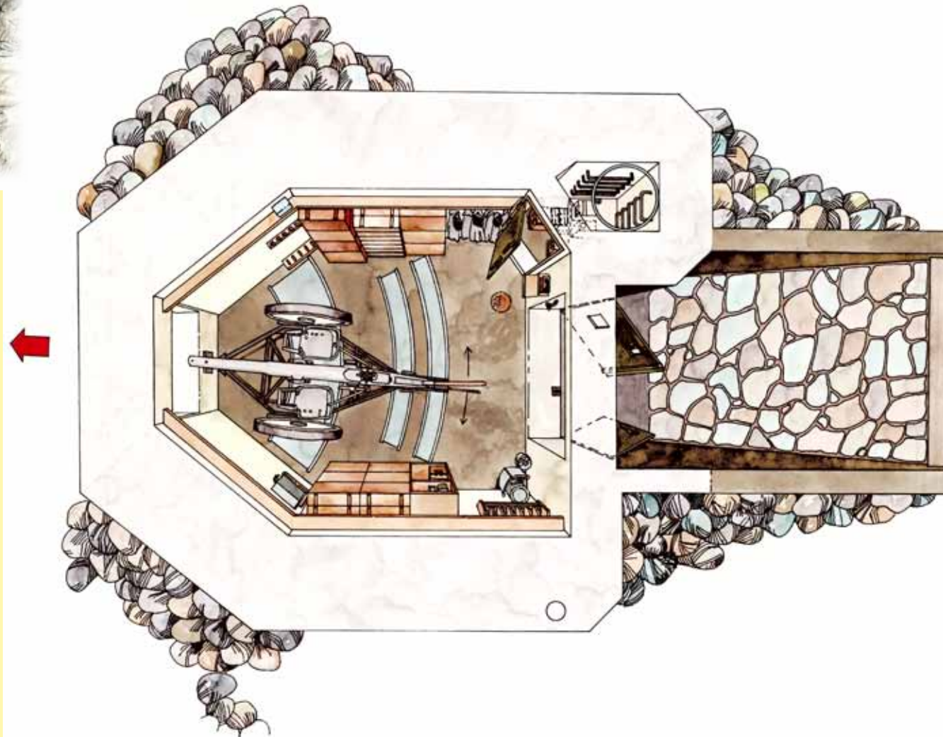
Kanon modell 1881 på plats i ett kanonvärn.
